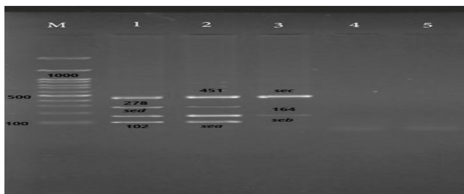
شکل ۳- تصویر PCR M: مارکر ۱۰۰ جفت بازی، چاهک‌های ۱-۲: نمونه‌های حاوی هر ۴ ژن ( sec (164bp) seb (164bp) sea (102bp) sed (278bp) و (451bp) چاهک ۳: ژن‌های sec (451bp) و seb (164bp) ، چاهک ۴: کنترل منفی.
