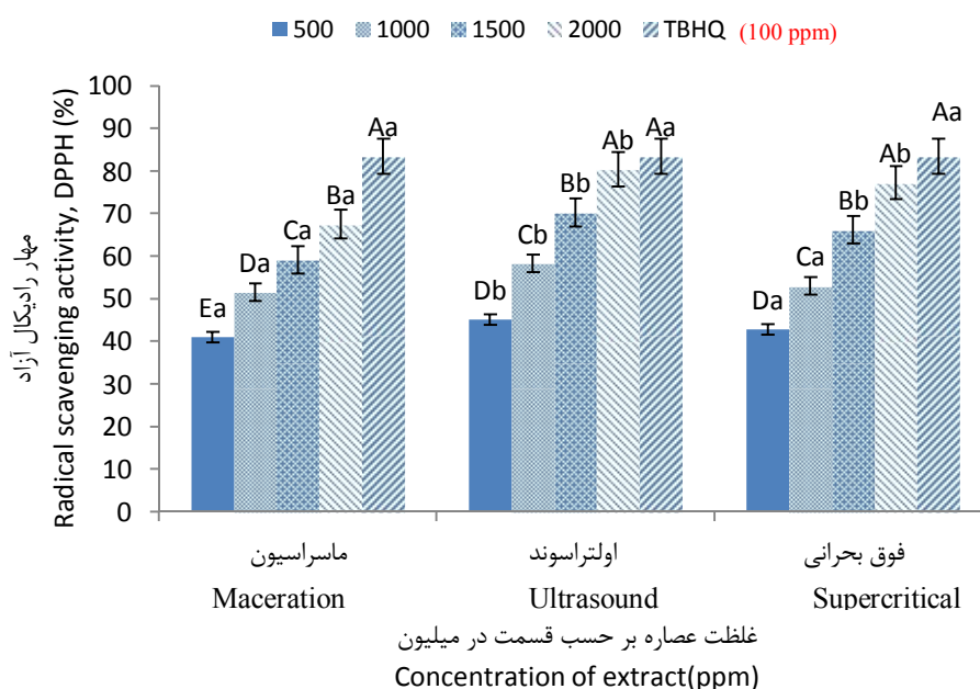
شکل ۲: فعالیت مهار رادیکال آزاد DPPH Figure 2. DPPH radical scavenging activity
